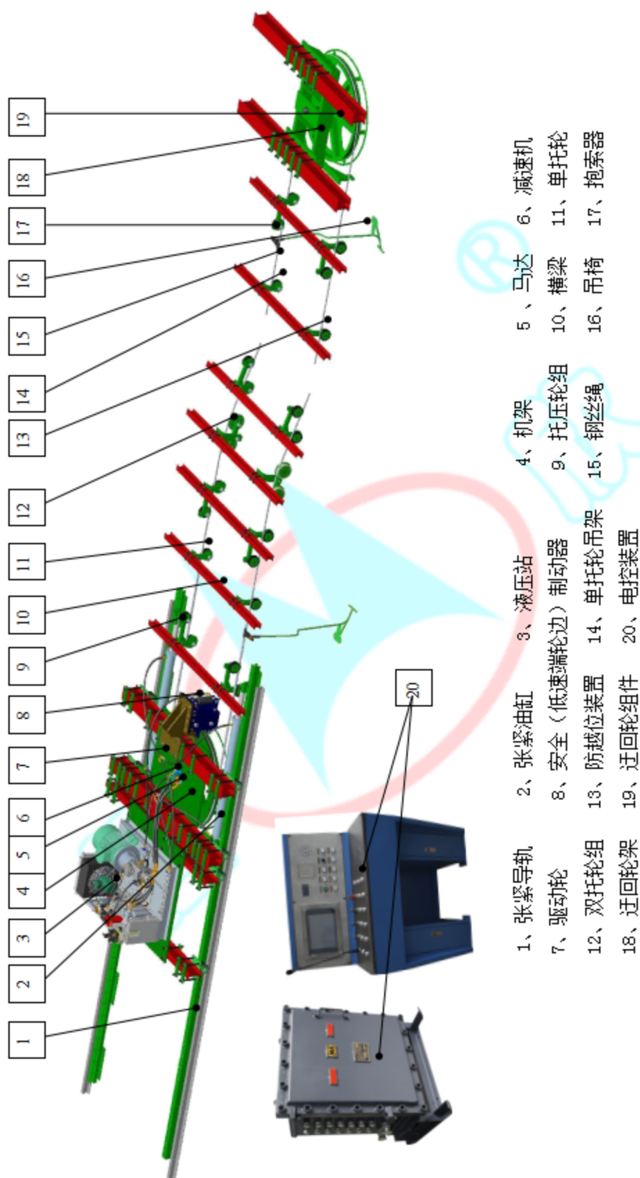
图 2-4 单轮驱动机头液压张紧架空式安装图 (单泵)
